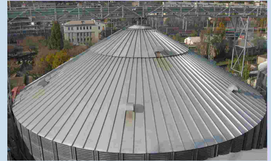
W-образное ребро жесткости, кольца для ветровой нагрузки и волнистая конструкция боковых стен зернохранилища
