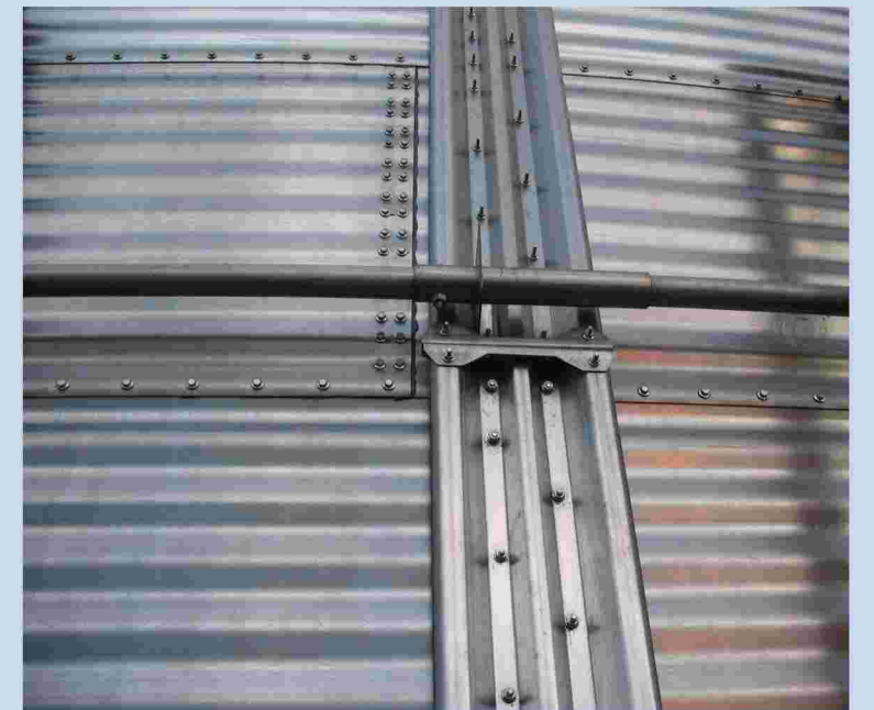
Конструкция крыши зернохранилища
