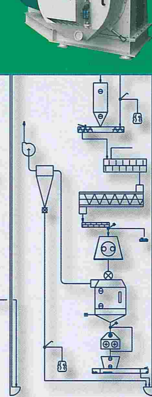
PELLETING / ГРАНУЛИРОВАНИЕ HEAT TREATMENT SECTION 1/ ТЕПЛООБРАБОТКА СЕКЦИЯ 1
