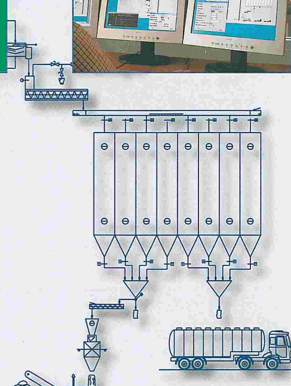
BAGGING OFF/ ОТГРУЗКА В МЕШКИ
