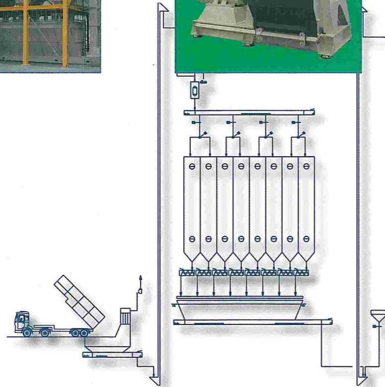
RECEPTION BULK/ ПРИЕМ СЫПУЧЕГО СЫРЬЯ
